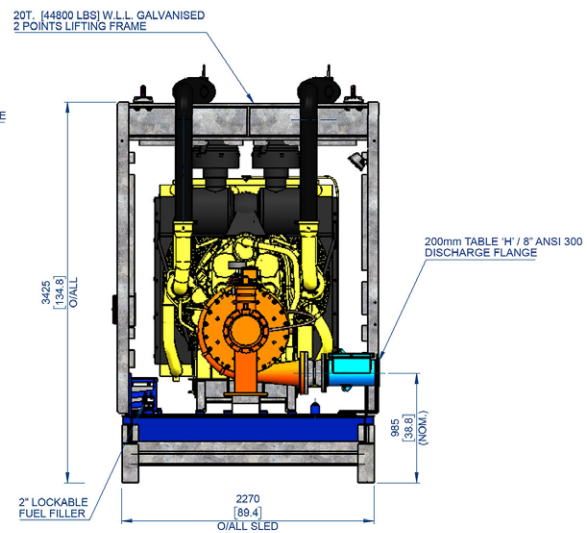
END ELEVATION
