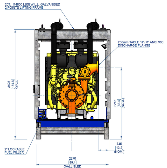
END ELEVATION
