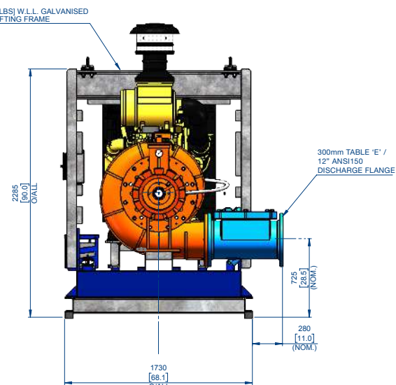
END ELEVATION
