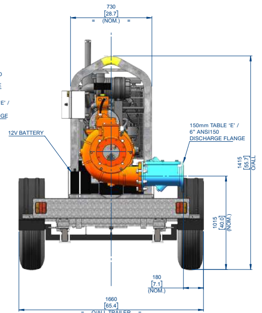
END ELEVATION
