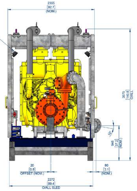
END ELEVATION
