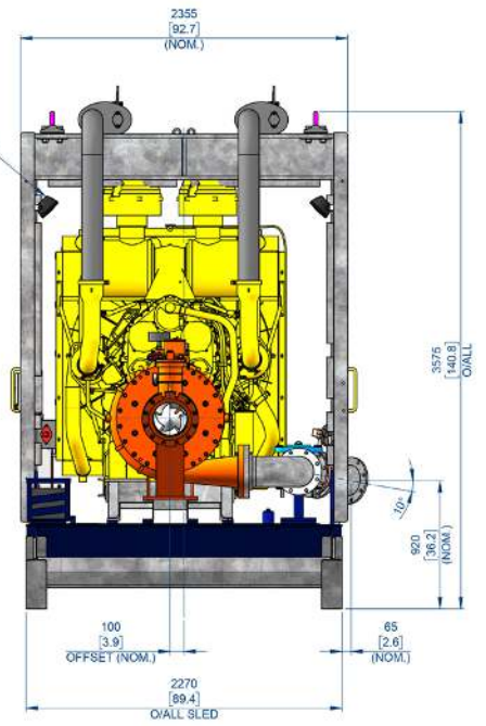
END ELEVATION
