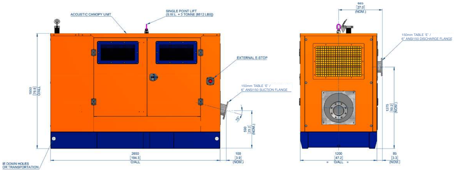
ELEVATION
